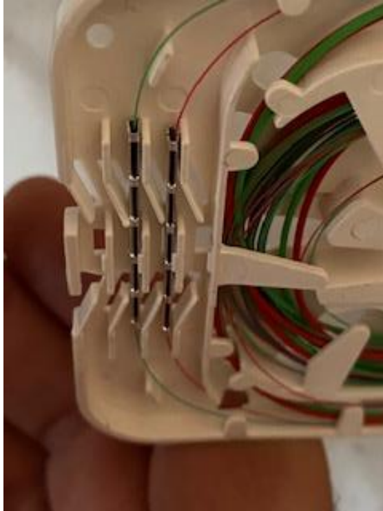
10. Spleißschutz ablegen
