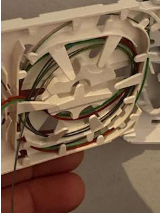
9. Faser einlegen
